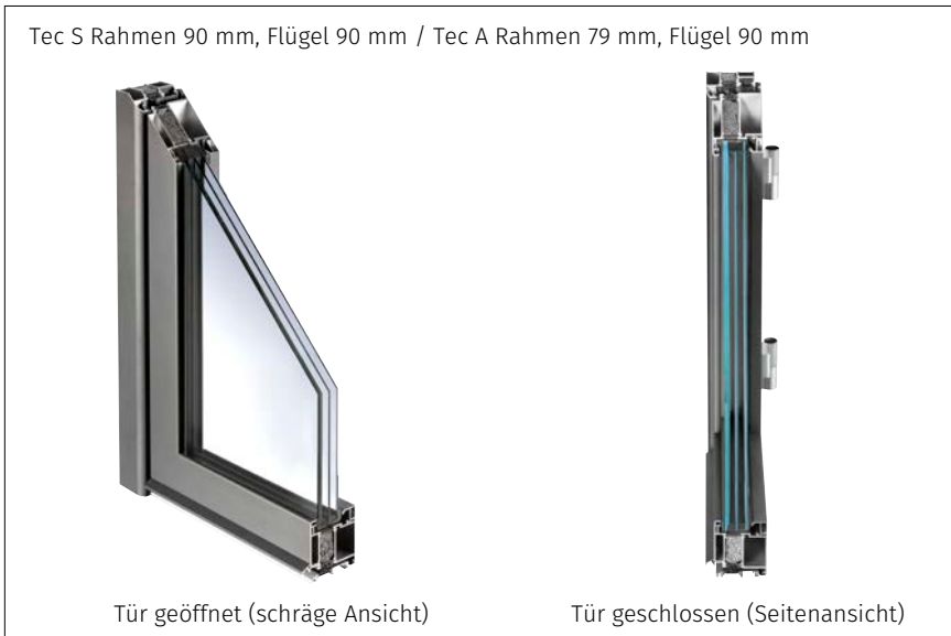
Tec A (Türrahmen bündig mit Flügelprofil)
